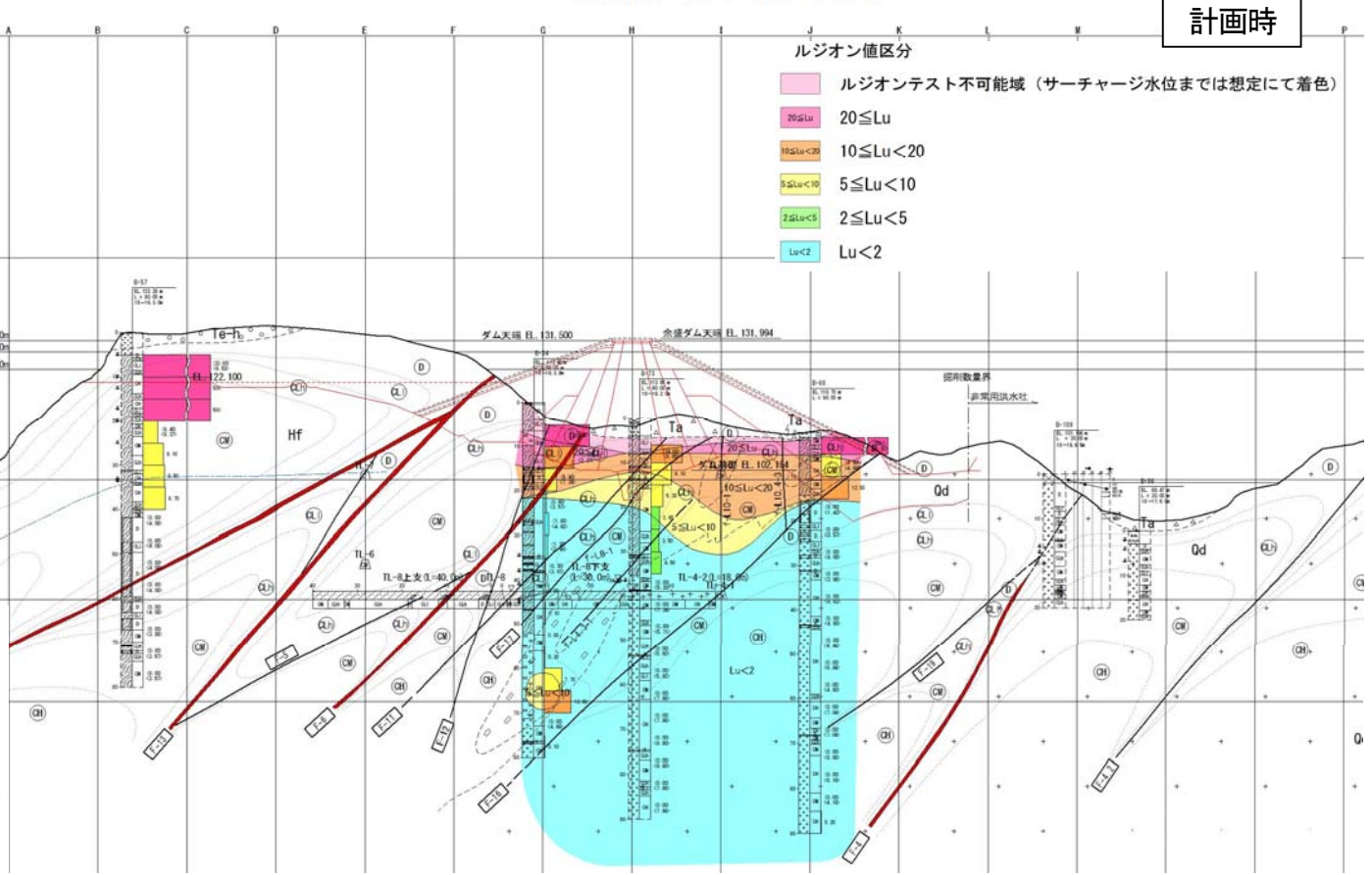
18測線 岩盤透水性区分図
