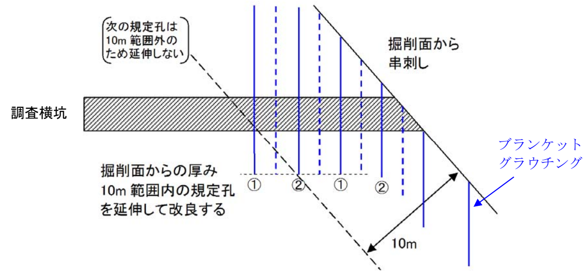
図-1 調査横坑に近接する箇所への延伸
