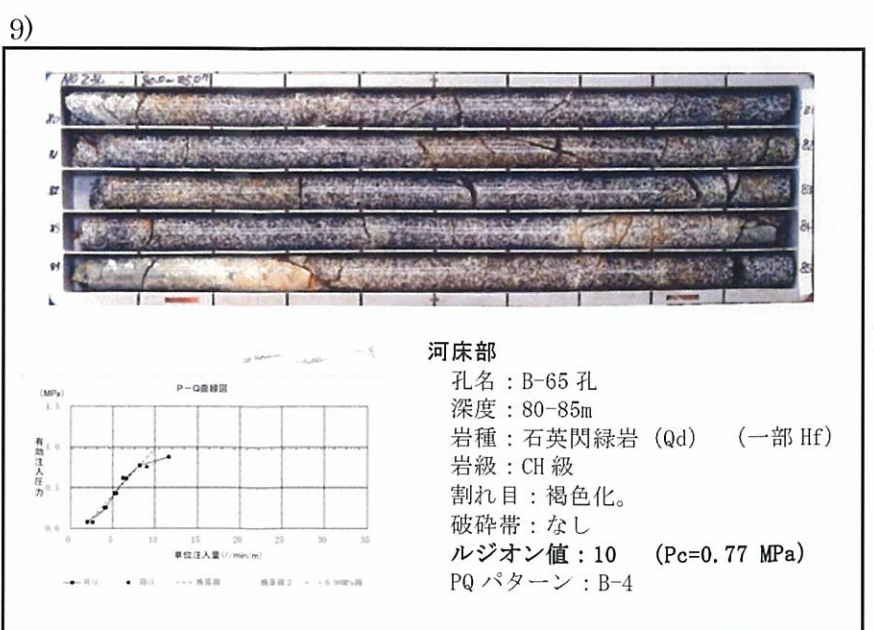
図-3.5.12 止水ラインにおける深部高透水箇所のパ-Q 曲線とコア状況①
