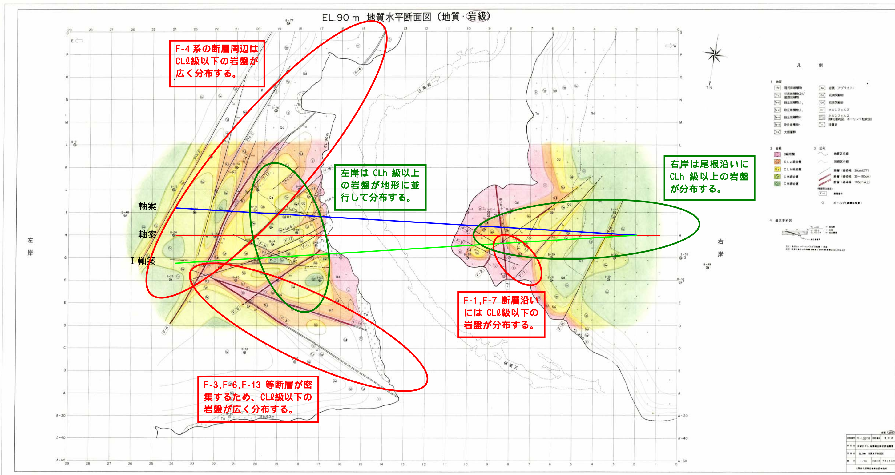
図-4.1.2 EL.90m 岩級スライス平面図
