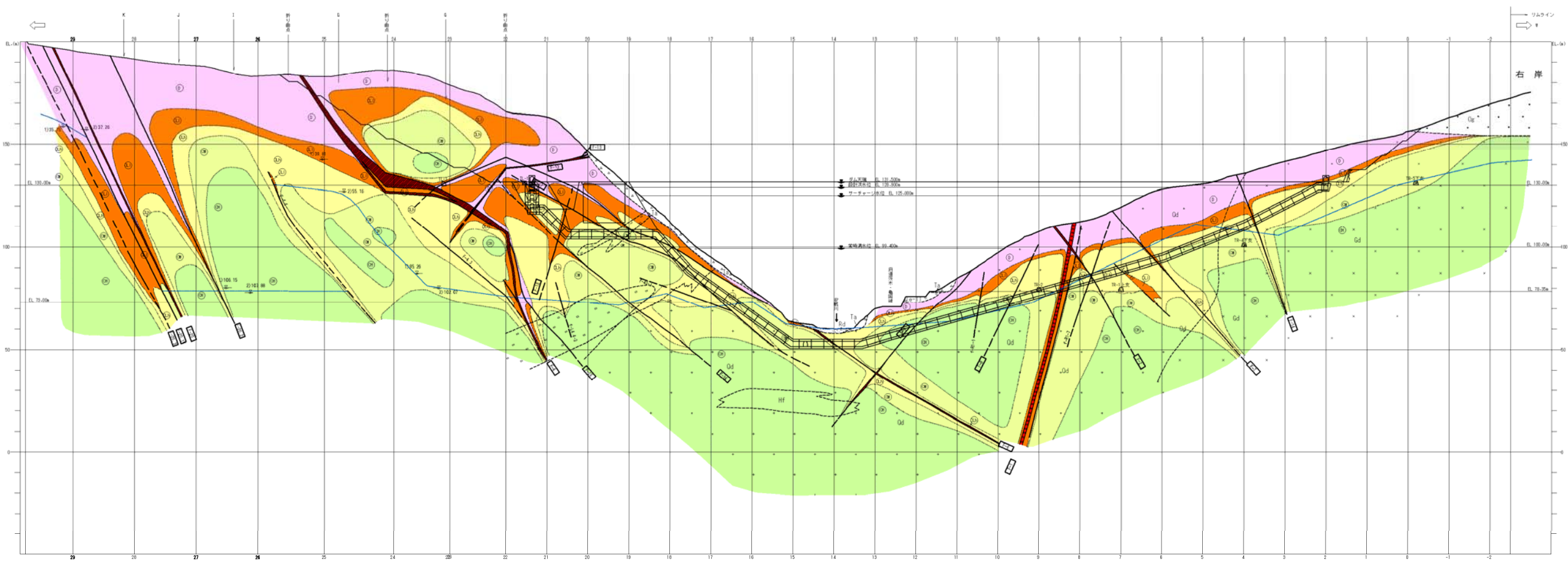
図 - 4.4.2 ダム軸縦断掘削形状
