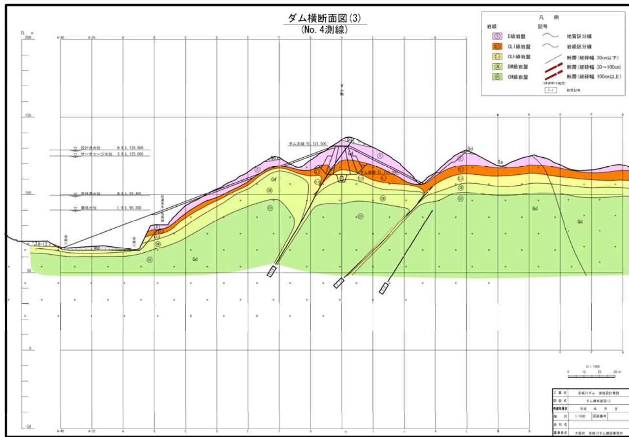
図 - 4.4.4 (1) ダム横断面図
