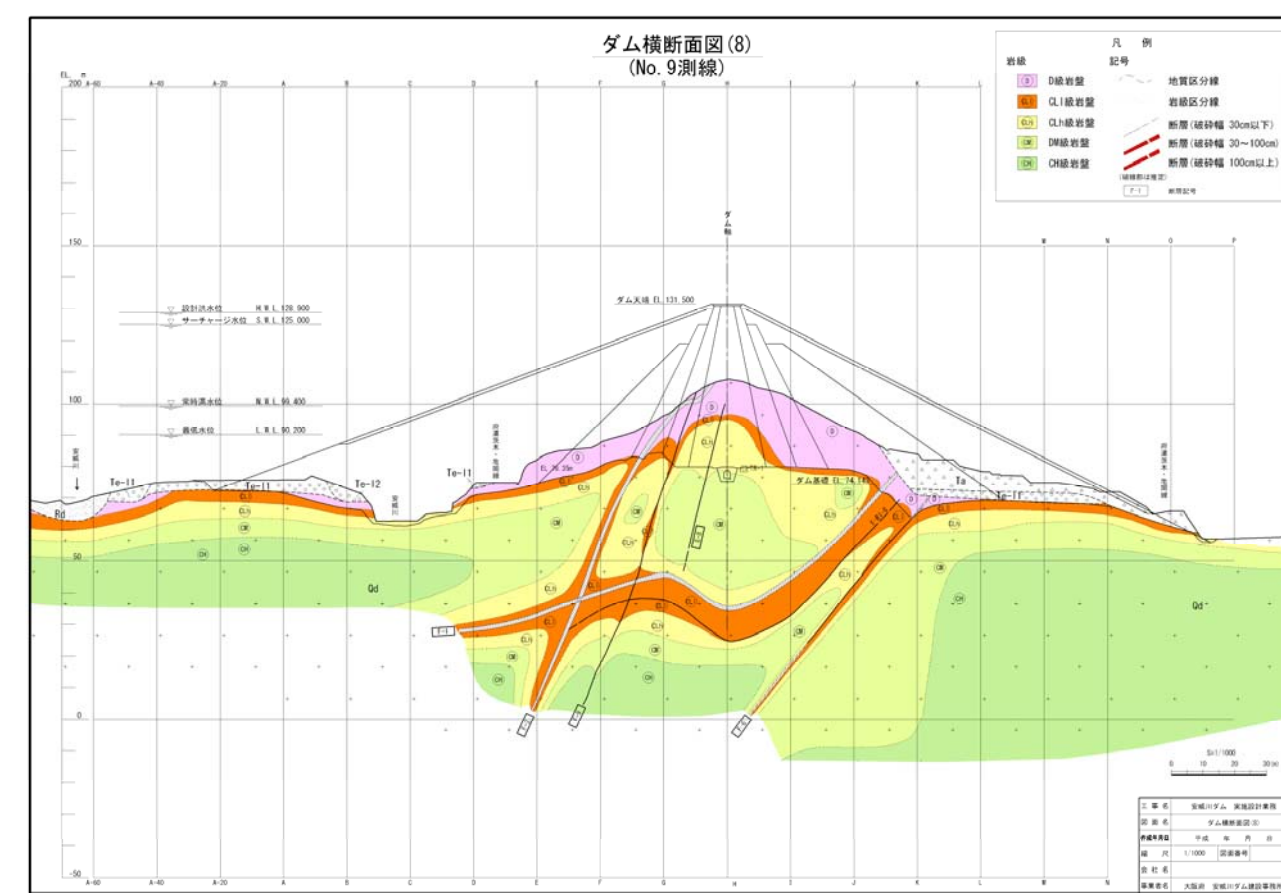
図 - 4.4.4 (2) ダム横断面図
