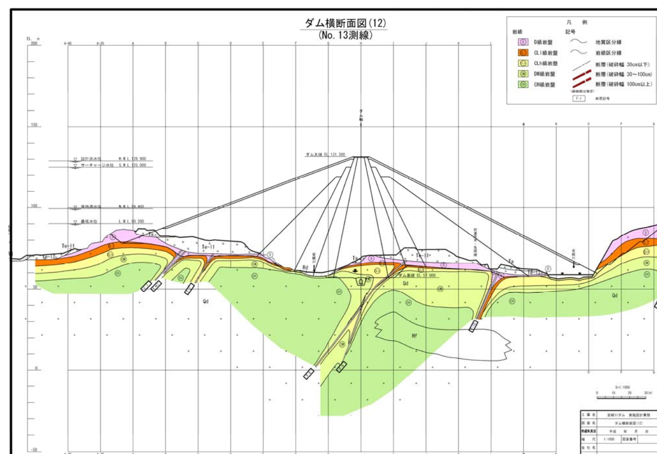
図 - 4.4.4 (3) ダム横断面図
