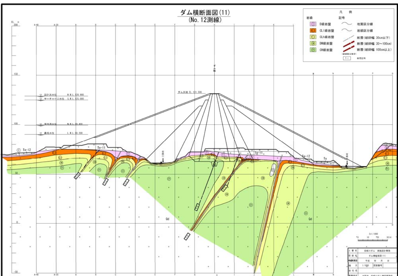
図 - 4.4.4 (3) ダム横断面図
