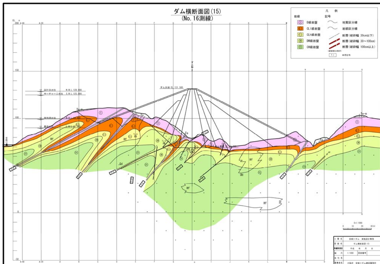
図 - 4.4.4 (4) ダム横断面図
