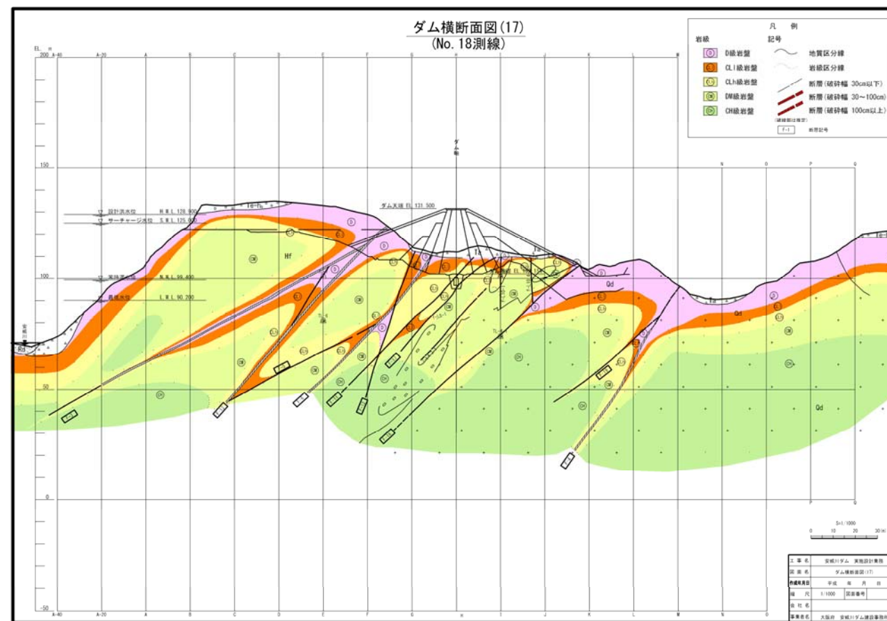
図 - 4.4.4 (5) ダム横断面図
