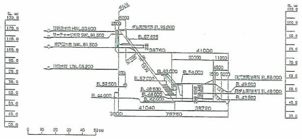
越流標準断面図
