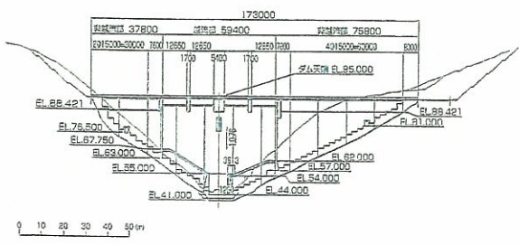
堤体下流断面図
